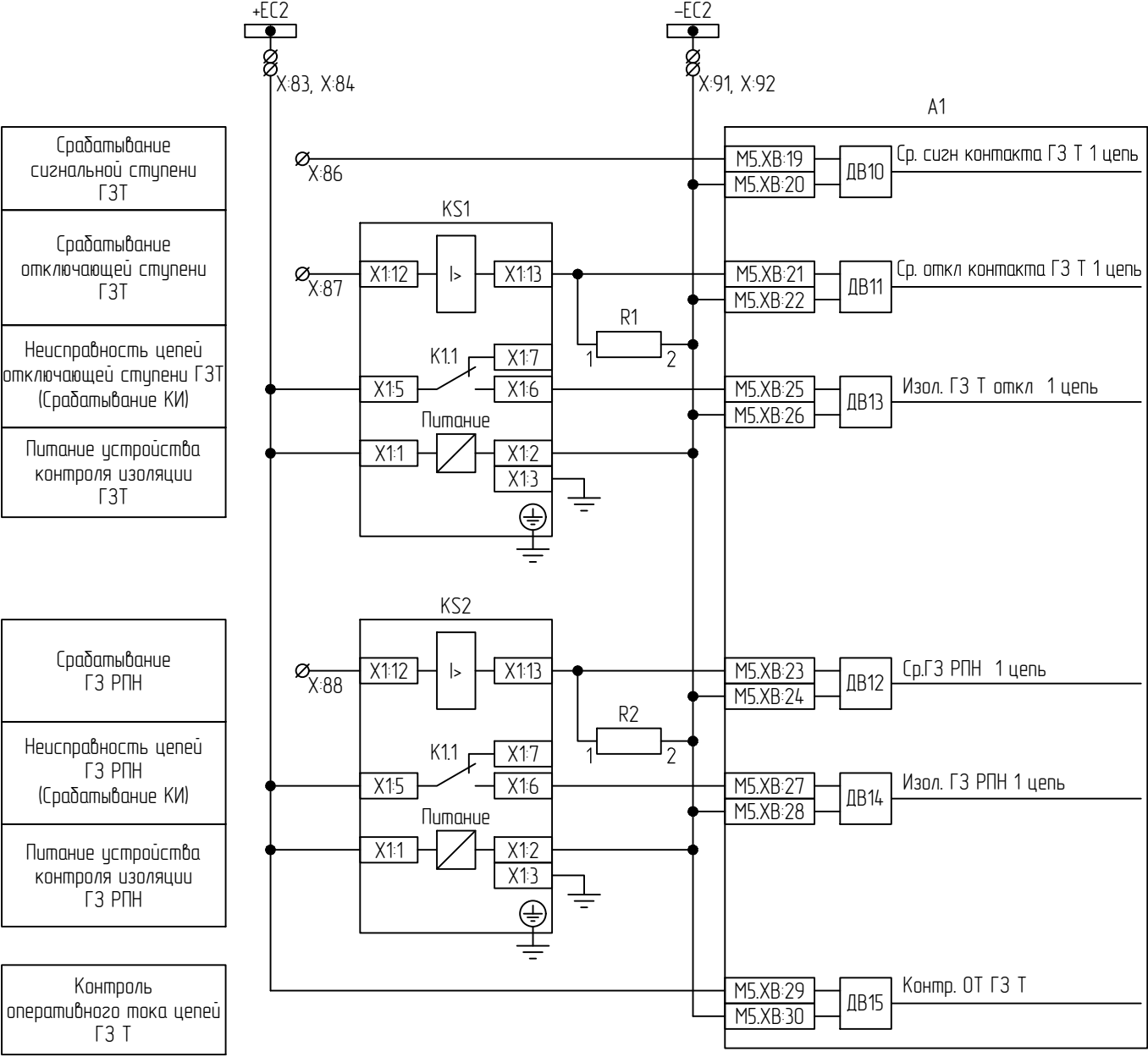
Цепи оперативного тока ГЗ Т А1
